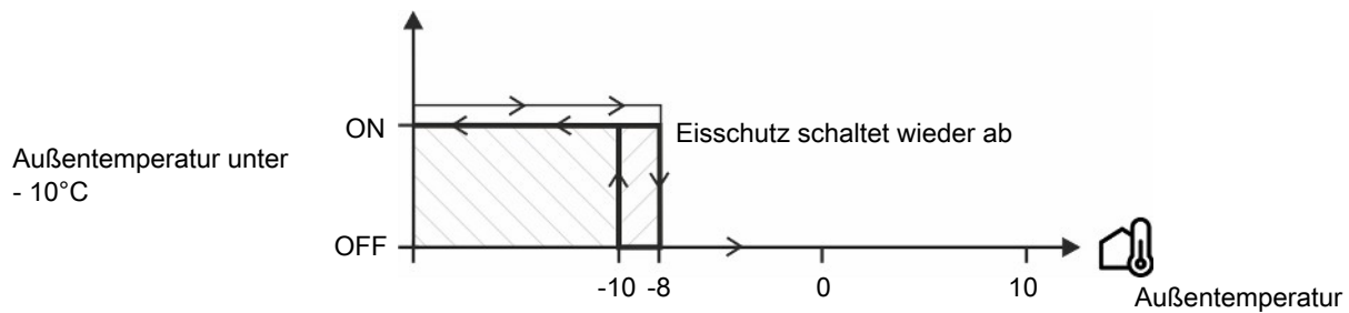
Abb. 16: Aktivierung von Eisschutz
