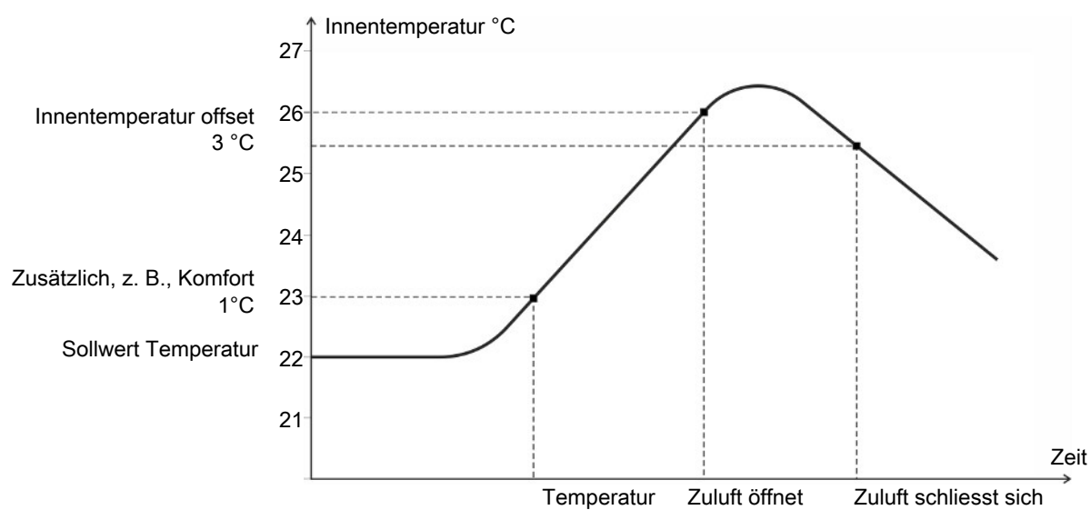
Abb. 9: Zuluft Combi-Diffus – Innentemperatur-geregelt
