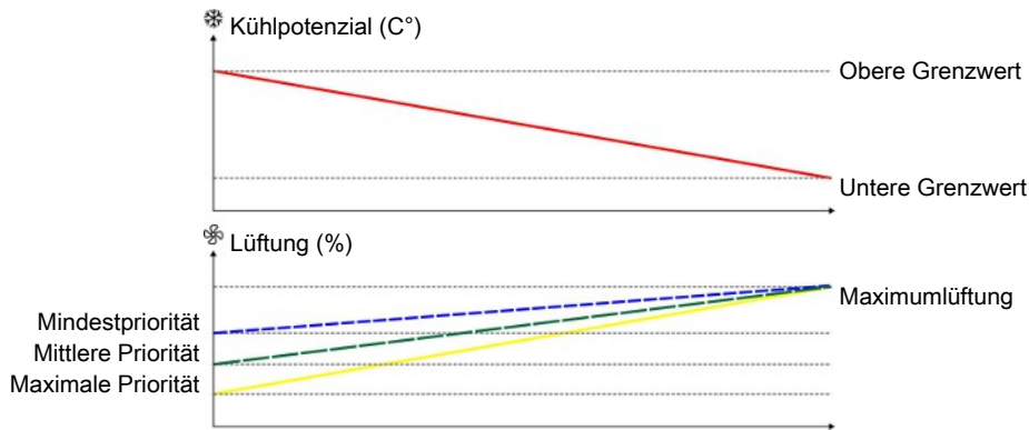
Abb. 28: Je höher das Kühlspotenzial, desto höher ist der frühe Start der Kühlung.
