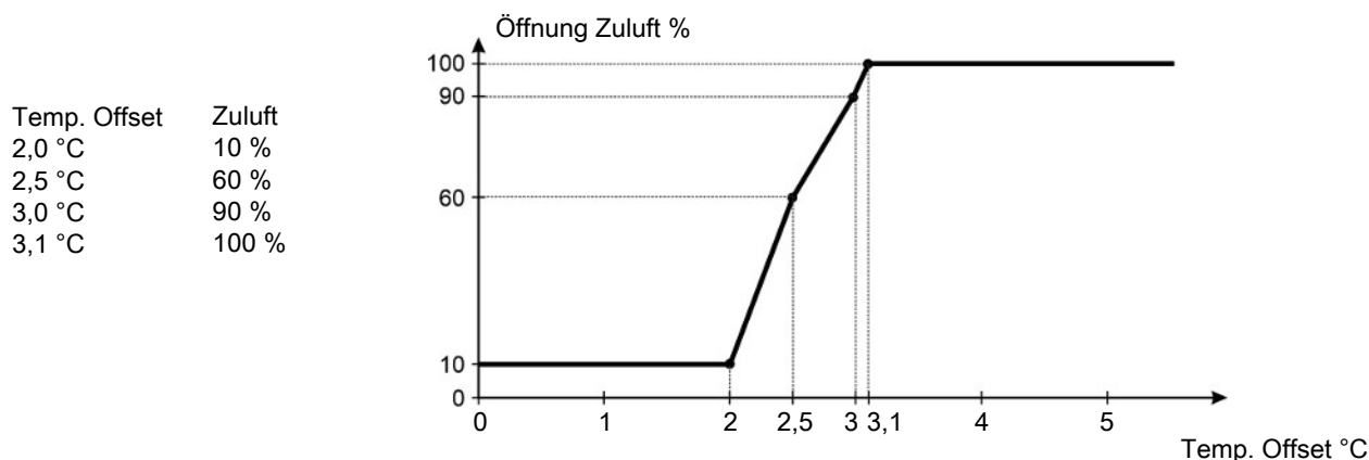
Abb. 11: Zuluft Combi-Diffus – stufenlose Öffnung basierend auf Innen- und Außentemperatur
