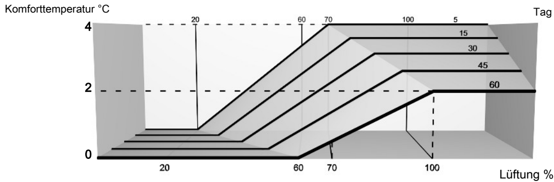
Abb. 5: Komforttemperatur bei dem Mast Produktion
