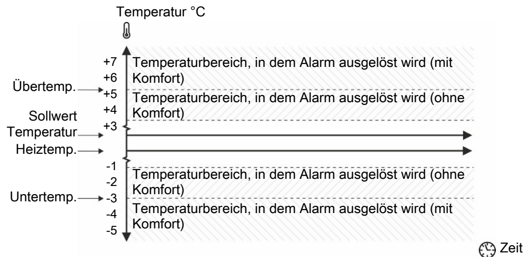
Abb. 41: Alarm für Übertemperatur und Untertemperatur
