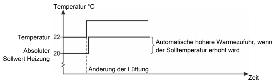
Abb. 34: Wärmezufuhr
