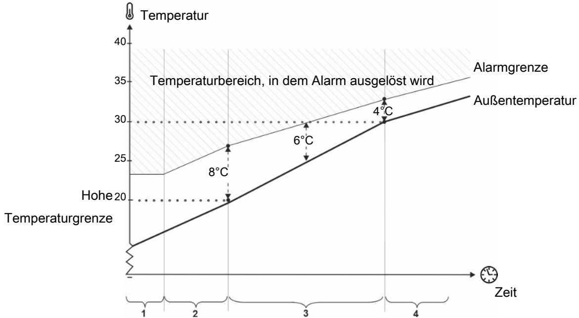
Abb. 42: Sommertemperatur bei 20 °C und 30 °C außen
