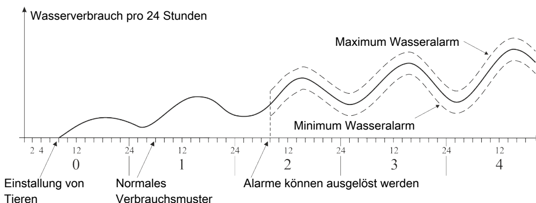
Abb. 43: Beispiel: Minimum und Maximum Wasseralarm
