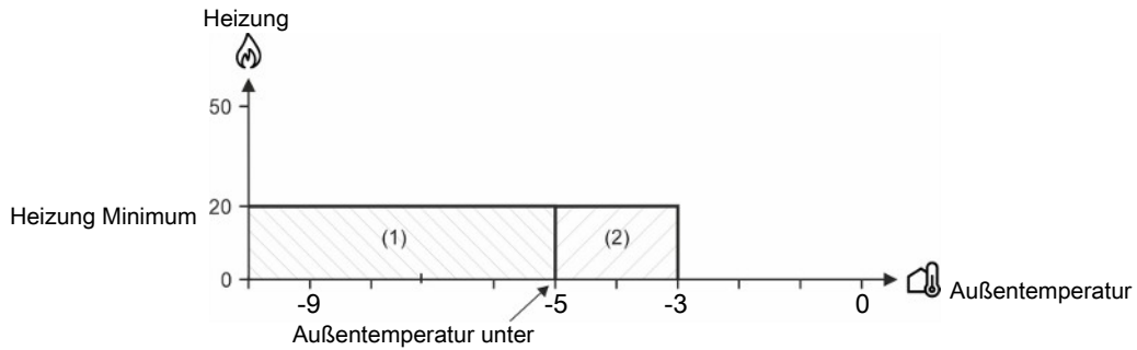
Abb. 35: Minimale Heizung bei sinkenden oder steigenden Außentemperaturen
