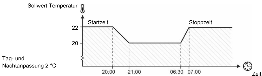
Abb. 7: Tag-Nacht-Anpassung als nächtliche Temperatursenkung.
