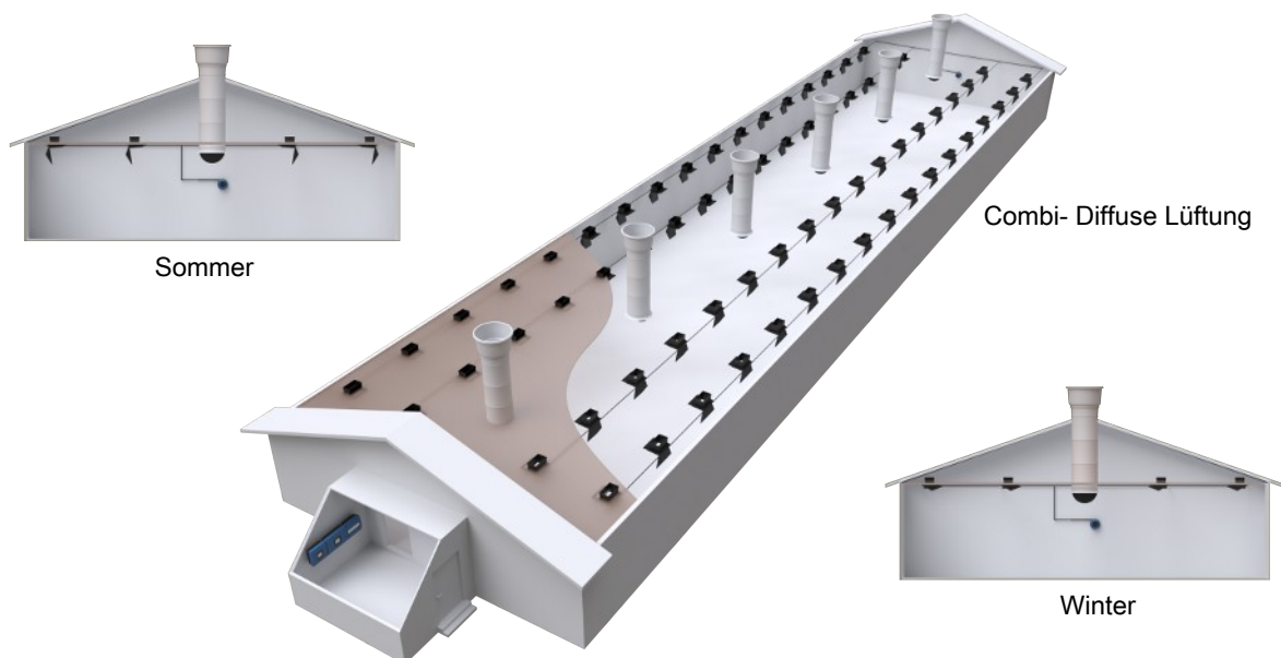
Abb. 8: Die Combi-Diffuse-Lüftung kombiniert die besten Eigenschaften der Lüftungssysteme: Diffus und LPV.
