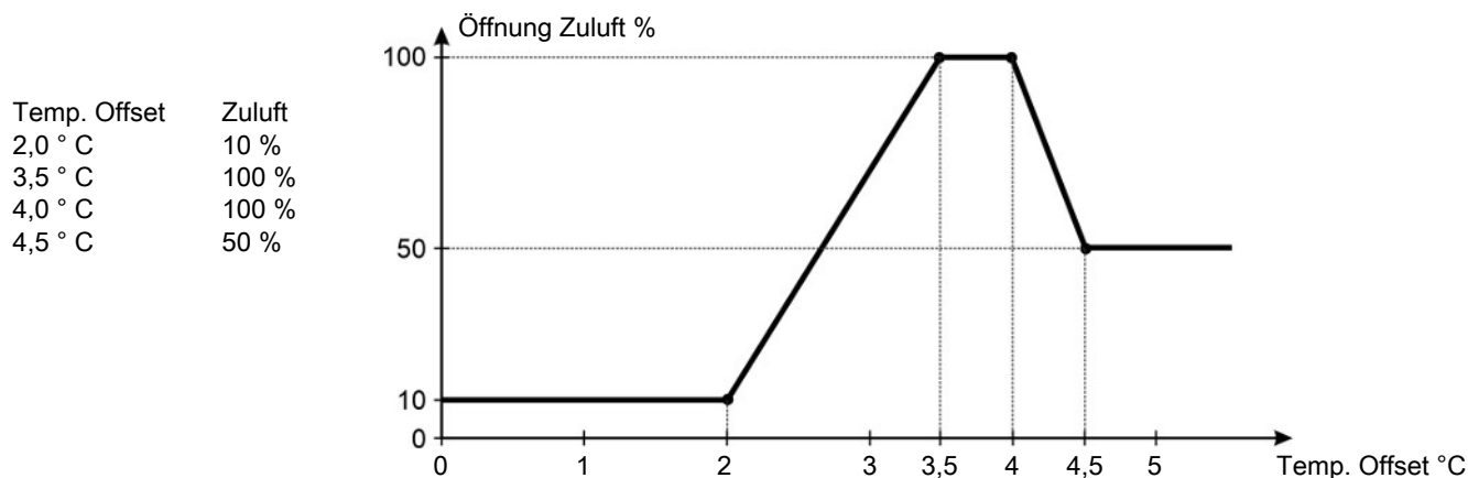
Abb. 10: Zuluft Combi-Diffus – verringerte stufenlose Öffnung bei hoher Außentemperatur
