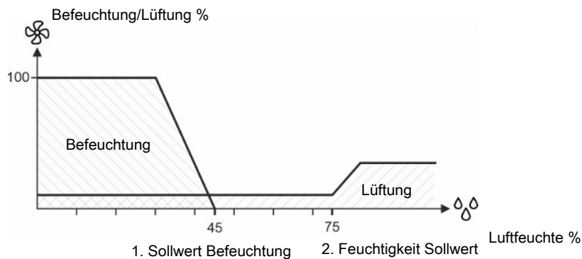
Abb. 12: 1. Abnehmende Luftfeuchtigkeit. Die Luftfeuchtigkeit liegt unter dem Sollwert Befeuchtung. Befeuchtung wird gestartet. 2. Zunehmende Luftfeuchtigkeit. Die Luftfeuchtigkeit liegt über dem Feuchtigkeitssollwert. Lüftung wird verstärkt.
