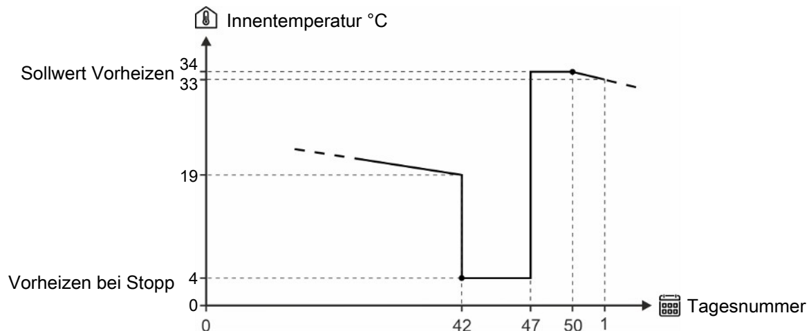
Abb. 38: Beispiel für Einstellung der Funktion Vorheizen.
