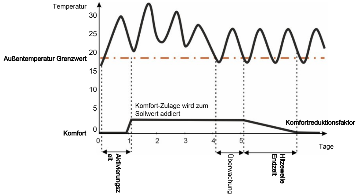
Abb. 4: Hitzewelle Komfort
