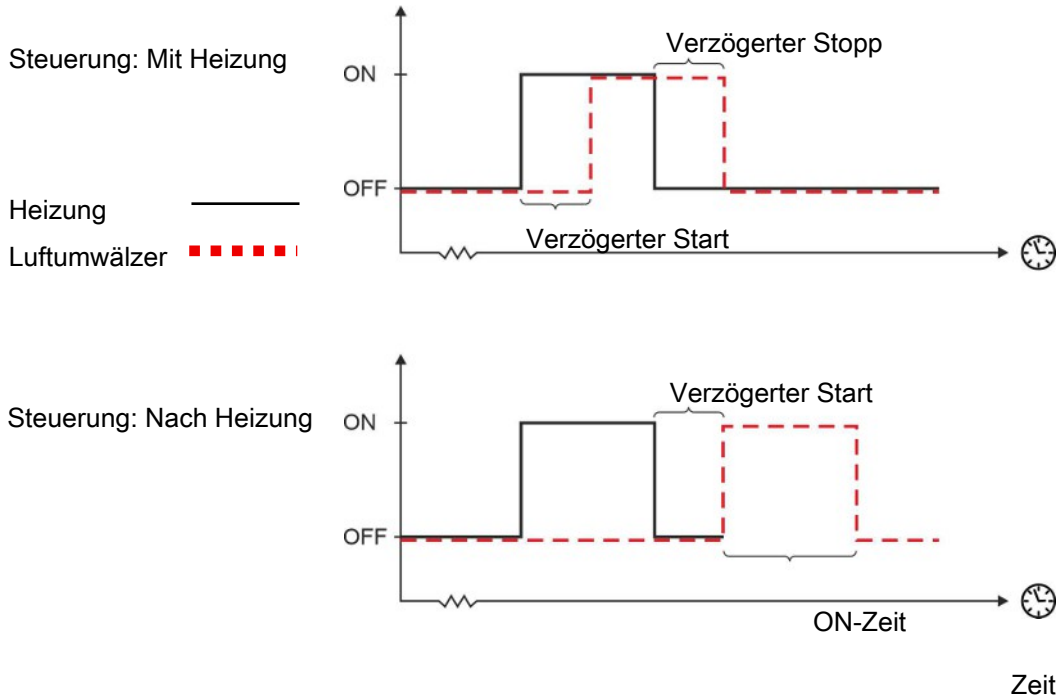
Abb. 25: Steuerung durch Heizquelle
