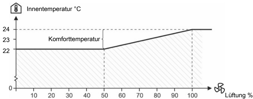
Abb. 6: Komforttemperatur bei kontinuierlichem Betrieb
