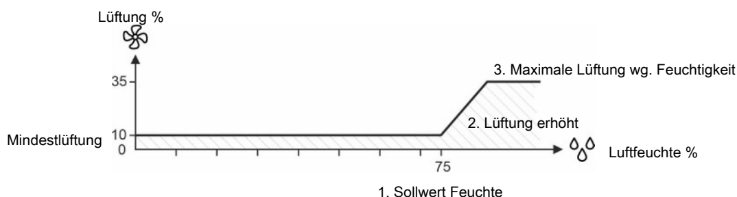
Abb. 14: Feuchtelüftung: 1. Die Luftfeuchtigkeit überschreitet den Feuchte-Sollwert. 2. Lüftung wird vom Stallcomputer verstärkt. 3. Steigerung bis zur maximalen Feuchtelüftung (35%).
